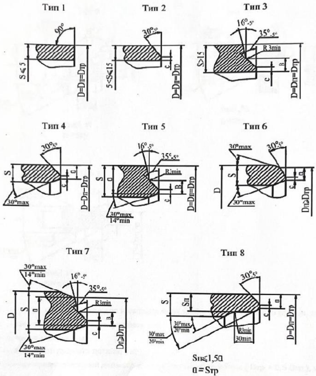
Рисунок 2, лист 1 – Варианты разделки кромок торцов детали
